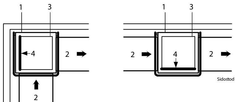
Placering av sidostöd
